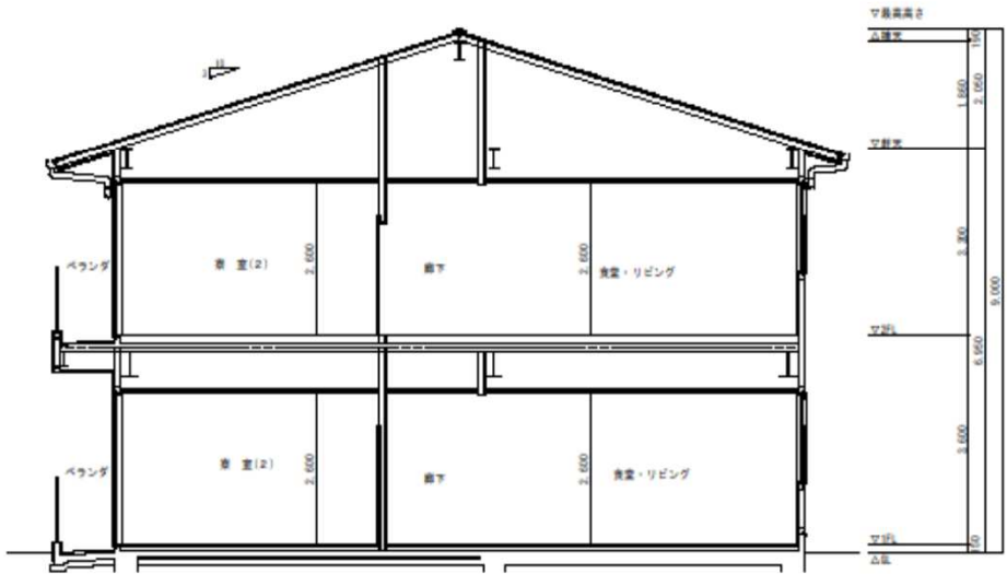
断面図
